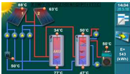
2 kol.polja / cijevni kol. / 1 sprem. PTV / 1 aku sprem / hidr.spjov pumpe / dogrijavanje kotao ulje/plin / recirkulacija PTV / mjerac protoka / osjetnik povratnog voda
