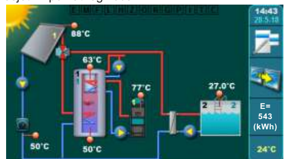
1 kol.polje / pločasti kol. / 1 aku s PTV / bazen / hidr.spjov zonski 3putni / dogrijavanje kotao na drva / recirkulacija PTV / mjerac protoka / osjetnik povratnog voda / osj. vanjske temperature
