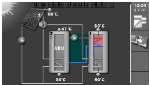
primjer: konfigurirano 2 spremnika, hidr. spoj: - Zonski 3-putni, Miješanje/dogrijavanje
