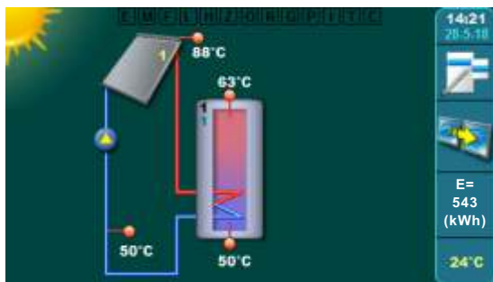
1 kol.polje / pločasti kol. / 1 sprem. PTV / osjetnik povratnog voda / osjetnik vanjske temperature
