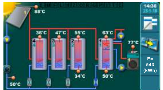
1 kol.polje / pločasti kol. / 4 sprem. PTV / hidr.spjov zonski 2putni / dogrijavanje kotao ulje/plin / recirkulacija PTV / mjerac protoka / osjetnik povratnog voda
